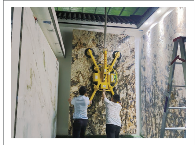
大理石室内搬运 直流八爪吸吊设备 HP-GX600-8S (600KG)
