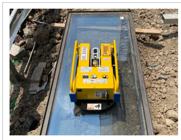
室外单元板块幕墙安装 直流单爪吸吊设备 HP-GI500-1S (500KG)
