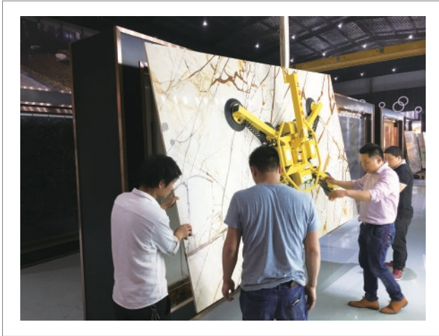
大理石室内搬运 直流八爪吸吊设备 HP-GX600-8S (600KG)
