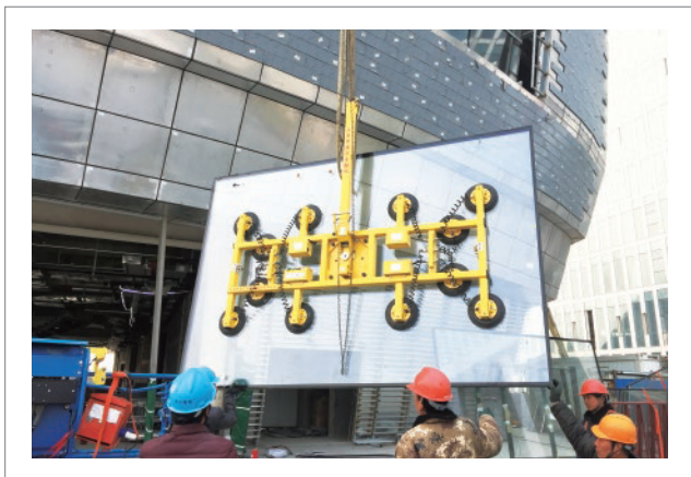
上海凯迪拉克中心幕墙安装 直流十二爪吸吊设备 HP-GH1200-12S (1200KG)
