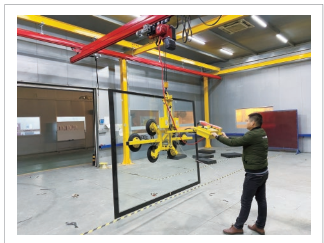
轨道幕墙玻璃搬运-葫芦升降 气动90度翻转 HP-GFD400-6S (400KG)
