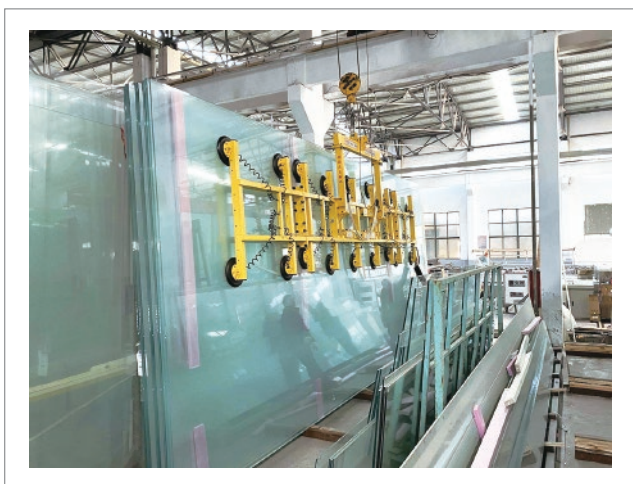
原片玻璃90度手动翻转搬运(双系统) 直流二十爪吸吊设备 HP-GH2000-20S (2000KG)
