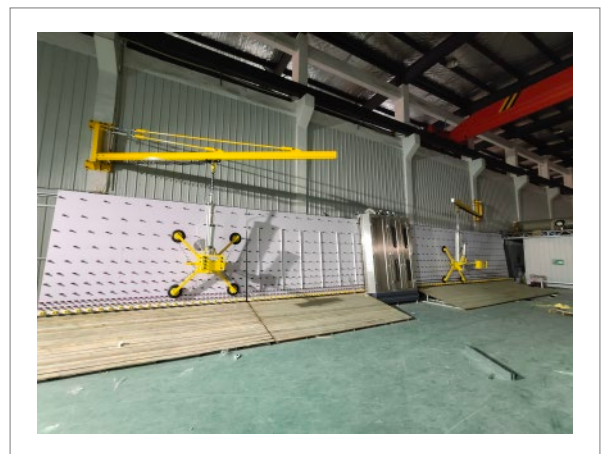
手动行走-手动摆臂 (KBK导轨) HP-QB500KG
