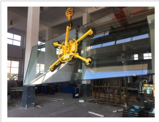
中空夹胶玻璃室内搬运 直流八爪吸吊设备 HP-GX600-8S (600KG)
