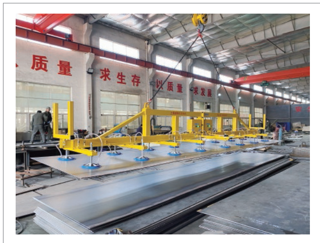
碳钢板水平搬运 (双系统) 直流十六爪吸吊设备 HP-BLZ3000-16S (3000KG)
